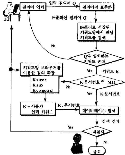
(그림 3-9) 키워드망을 이용한 정보검색 알고리즘 (Fig. 3-9) IR algorithm using keyword network
