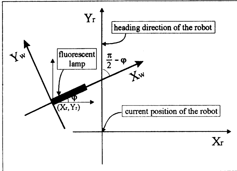
그림 9. 로봇 좌표계와 월드 좌표계간의 관계
